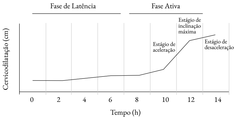
Figura 1: Curva Sigmóide de cervicodilatação (cm) das fases de latência e ativa e das divisões preparatórias de dilatação pélvica do trabalho de parto (Friedman, 1954) (DAVIM et al. #).
